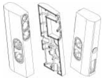
Computer gestütztes Gehäusedesign Computer aided cabinet design
